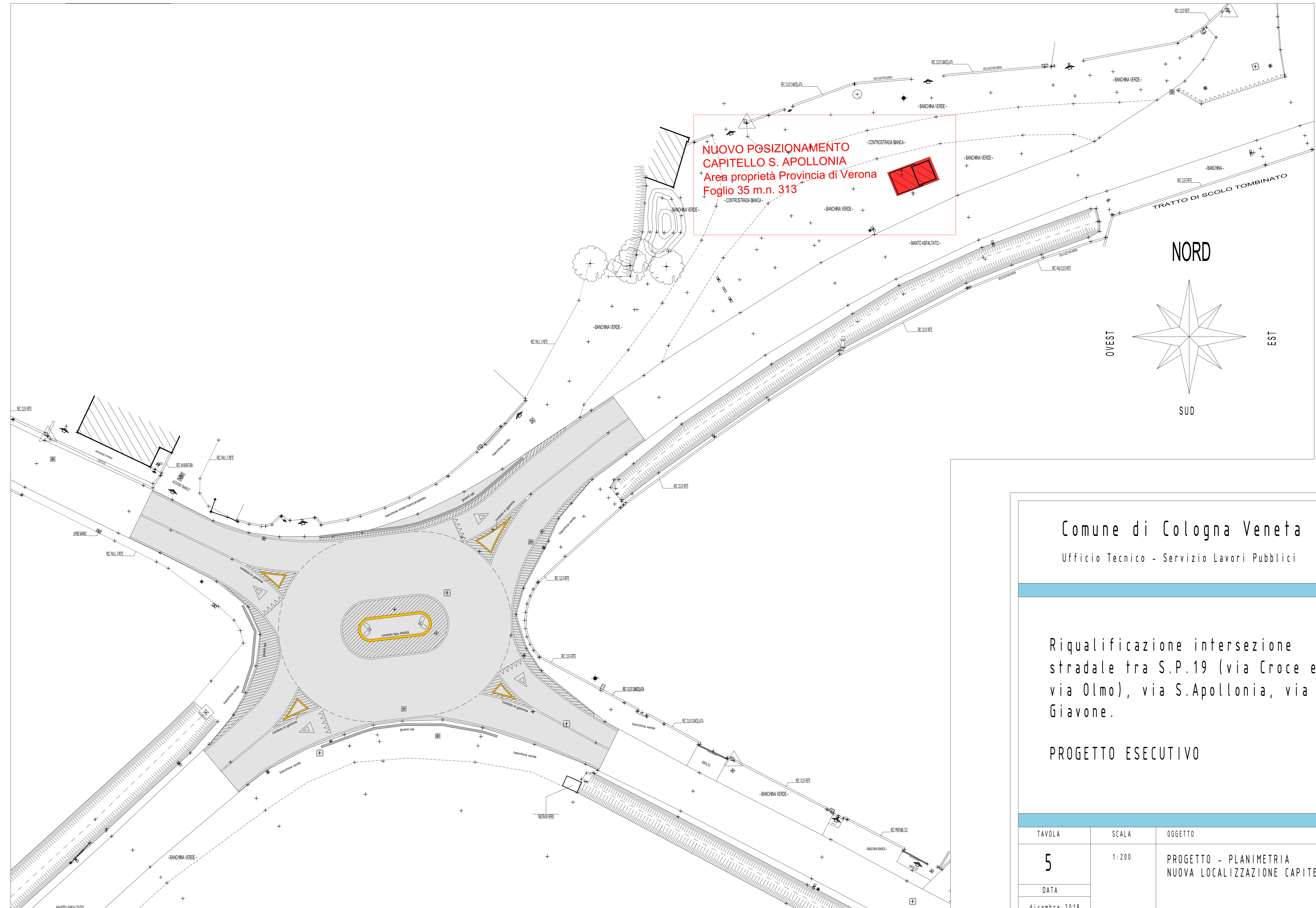
PROGETTO NUOVO POSIZIONAMENTO CAPITELLO PLANIMETRIA SCALA 1:200
